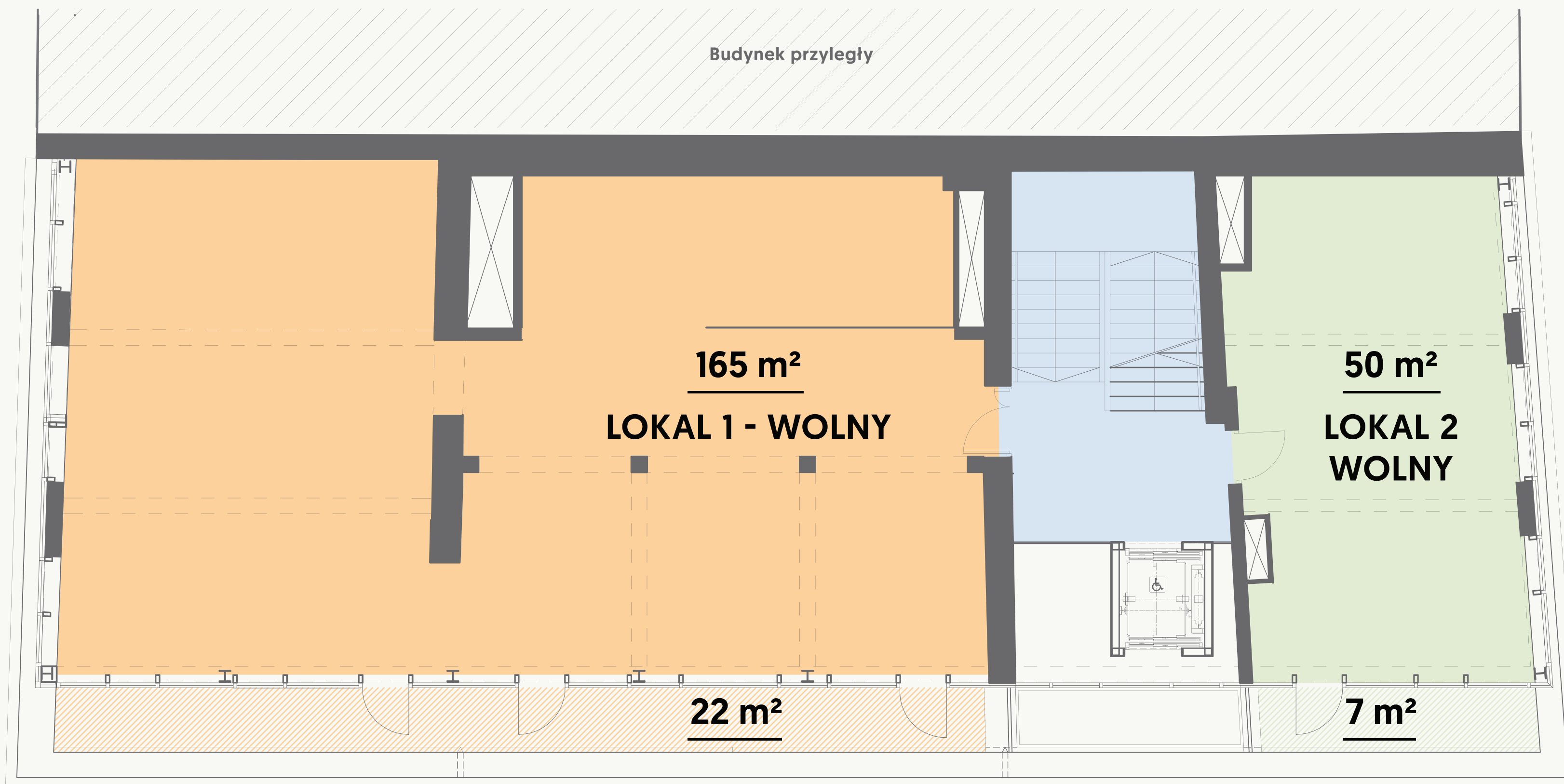
WARIANT I: RZUT POZIOMU +2
